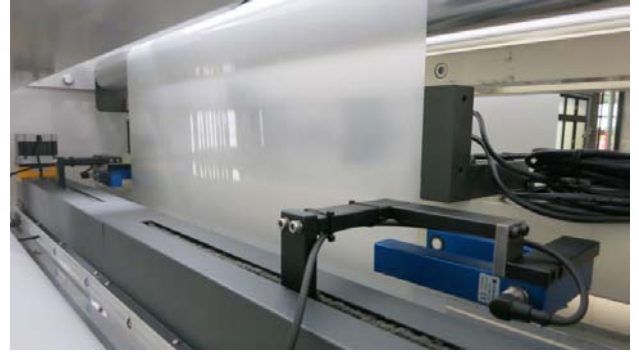
Otomatik Sensör Pozisyoner (ASP) üflemlerli film makinesi üzerinde kullanılmaktadır.
